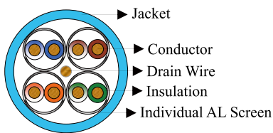
Cat7 U/FTP
